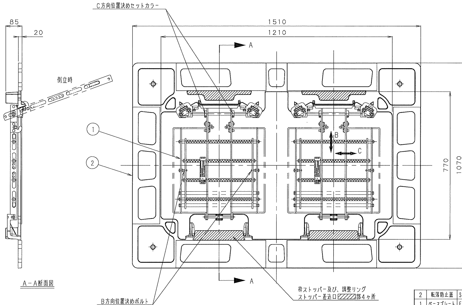
平面図
